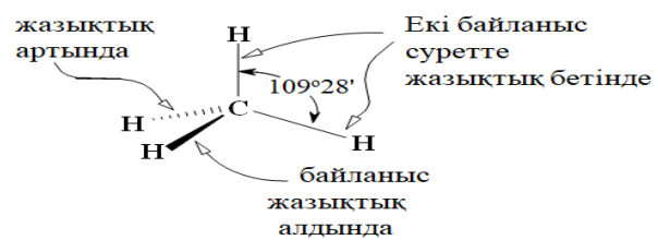
Стереохимиялық формуласы
